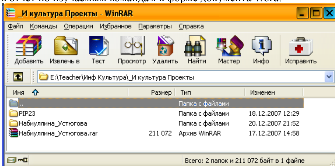
Рис.1. Архиватор WinRAR.
